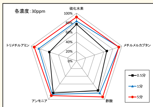
悪臭の除去率(シュカッターSR)
