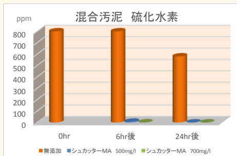
混合汚泥の消臭効果(シュカッター MA)
